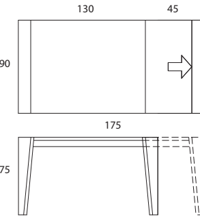
Cod. 558 / 042 L130+45 x P90 x H75 Tavolo allungabile / Extendible table / Table de repas extensible
