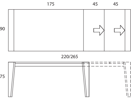
Cod. 558 / 046 L175+45+45xP90xH75 Tavolo allungabile / Extendible table / Table de repas extensible
