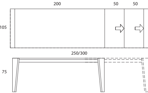
Cod. 658 / 048 L200+50+50xP105xH75 Tavolo allungabile / Extendible table / Table de repas extensible
