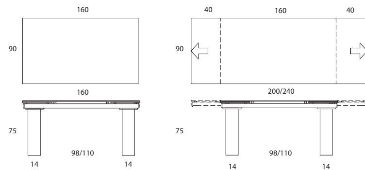
Cod. 380/382 L160 + 40 + 40 x P90 x H75 Tavolo allungabile / Extendible table / Table de repas extensible
