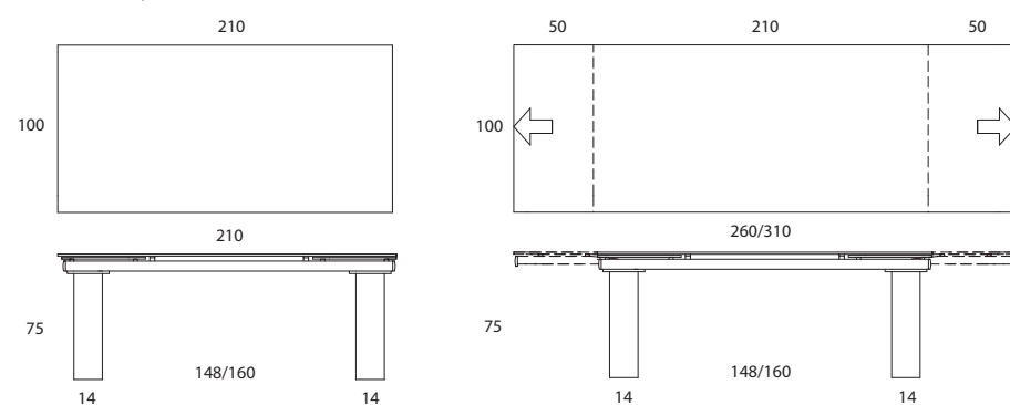
Cod. 380/382 L210 + 50 + 50 x P100 x H75 Tavolo allungabile / Extendible table / Table de repas extensible
